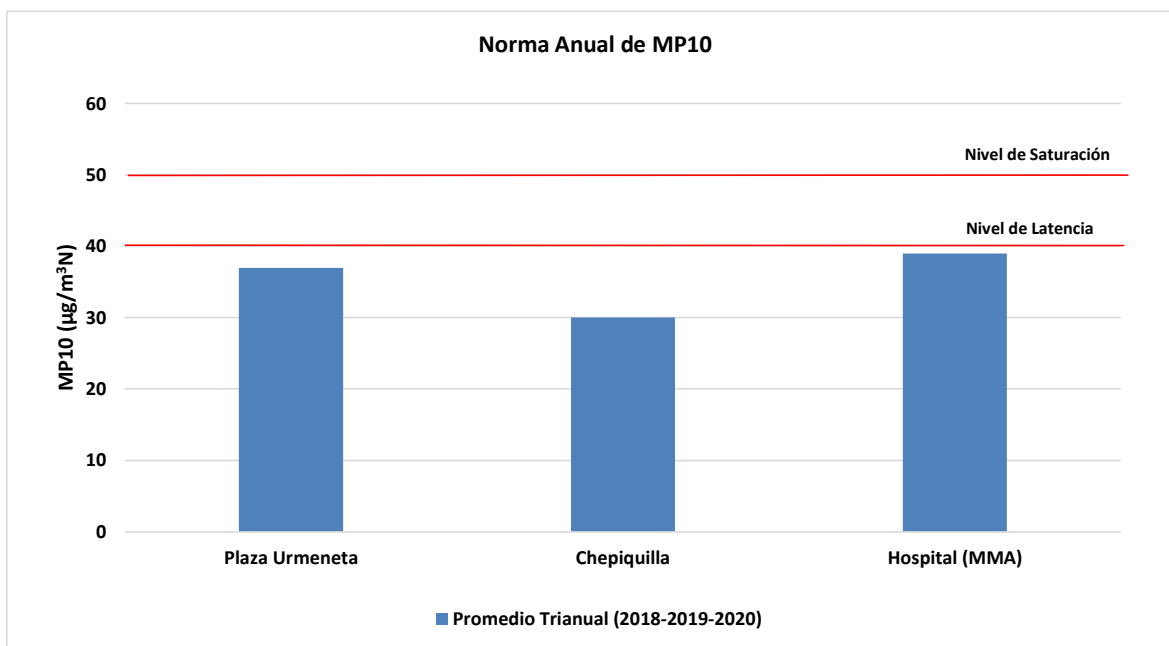
Gráfico 2 Norma Anual para MP10, Promedio trianual periodo 2018 al 2020
