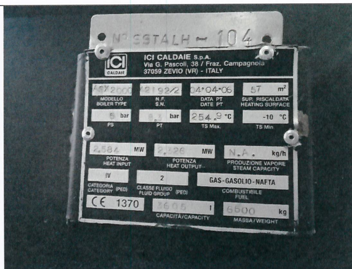
Fotografía 4. Placa de caldera Marca ICI Caldaie (N° Registro AS SSTATLH-104).
