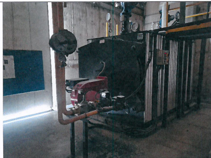
Fotografía 3. Caldera de planta Fanaloza, detenida al momento de la inspección.
