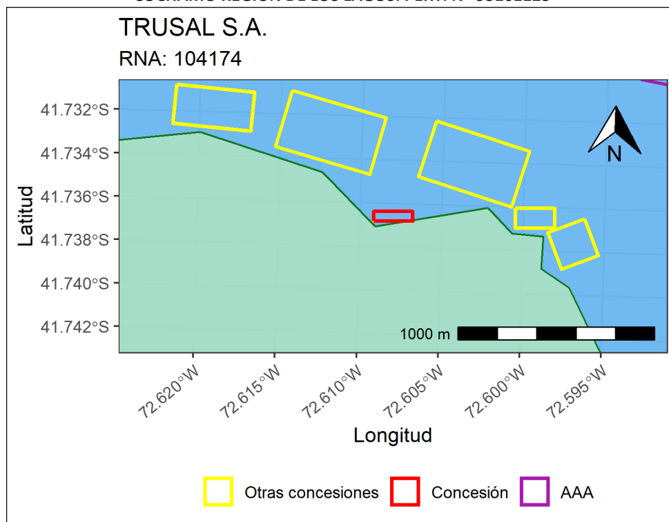
Figura 1. Ubicación UF CENTRO DE CULTIVO DE SALMONIDOS ESTERO RELONCAVI SECTOR BAHIA MARTIN COMUNA DE COCHAMO REGION DE LOS LAGOS. PERT. N° 93101123
