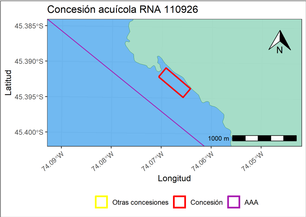
Figura 1. Ubicación UF CES JUD (RNA 110926)
