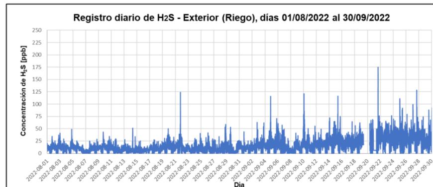
Figura N° 5. Diagrama de ácido sulhídrico ( H_2S ) – Exterior (riego) con respecto al tiempo.
