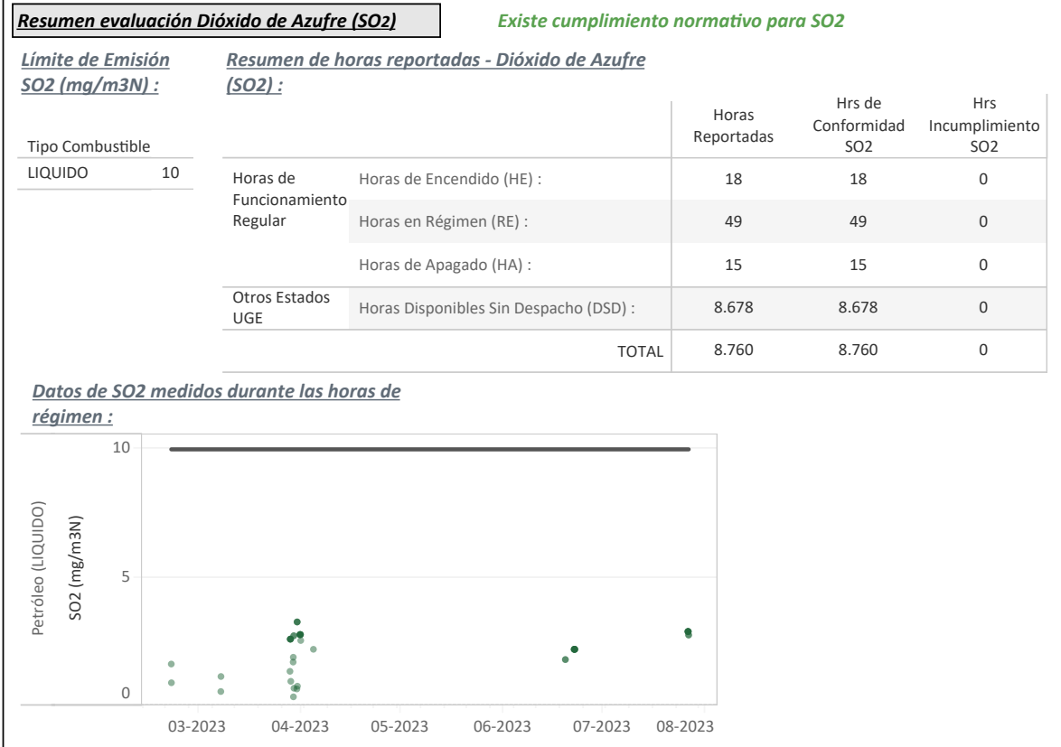
Figura N°2 - Resumen horas reportadas para Dióxido de Azufre (SO 2 ) - Año 2023
