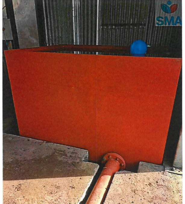
Estanque acumulador de agua sistema de abatimiento en plena capacidad (3 m3)
