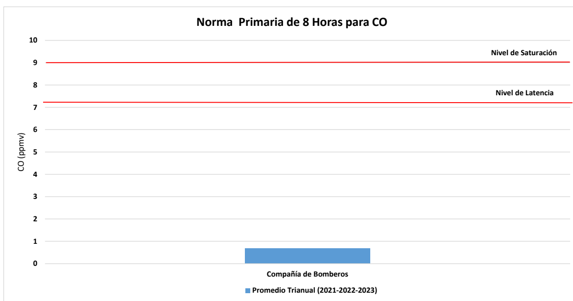
Gráfico 6 Norma 8 horas para CO, promedio trianual para el período 2021 al 2023
