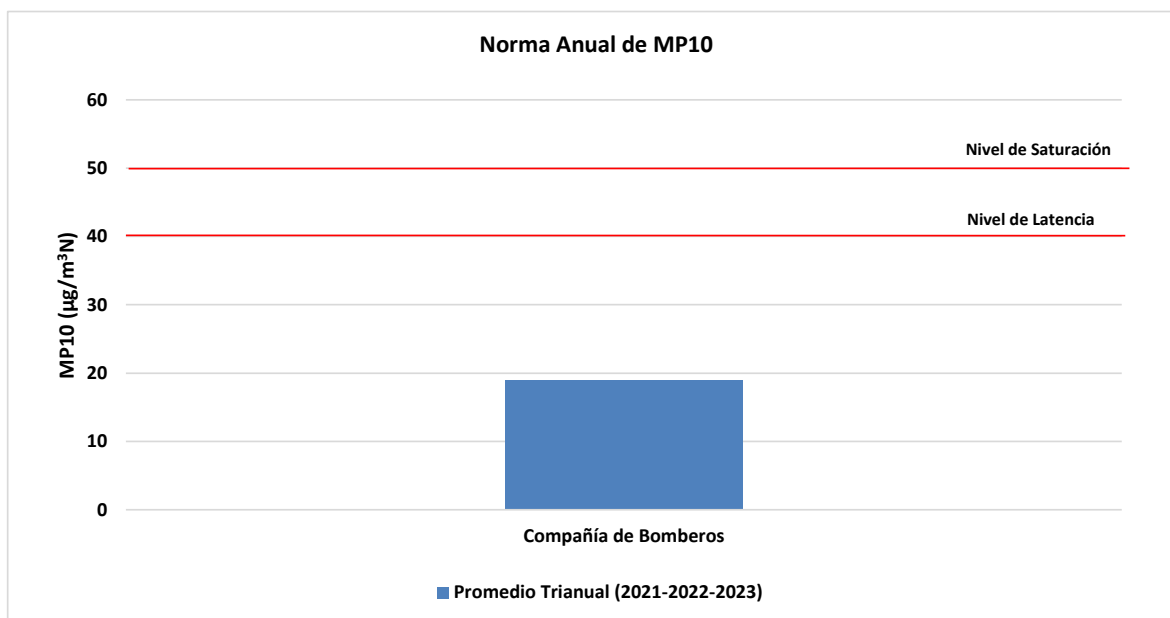
Gráfico 2 Norma anual para MP10 promedio trianual para el período 2021 al 2023
