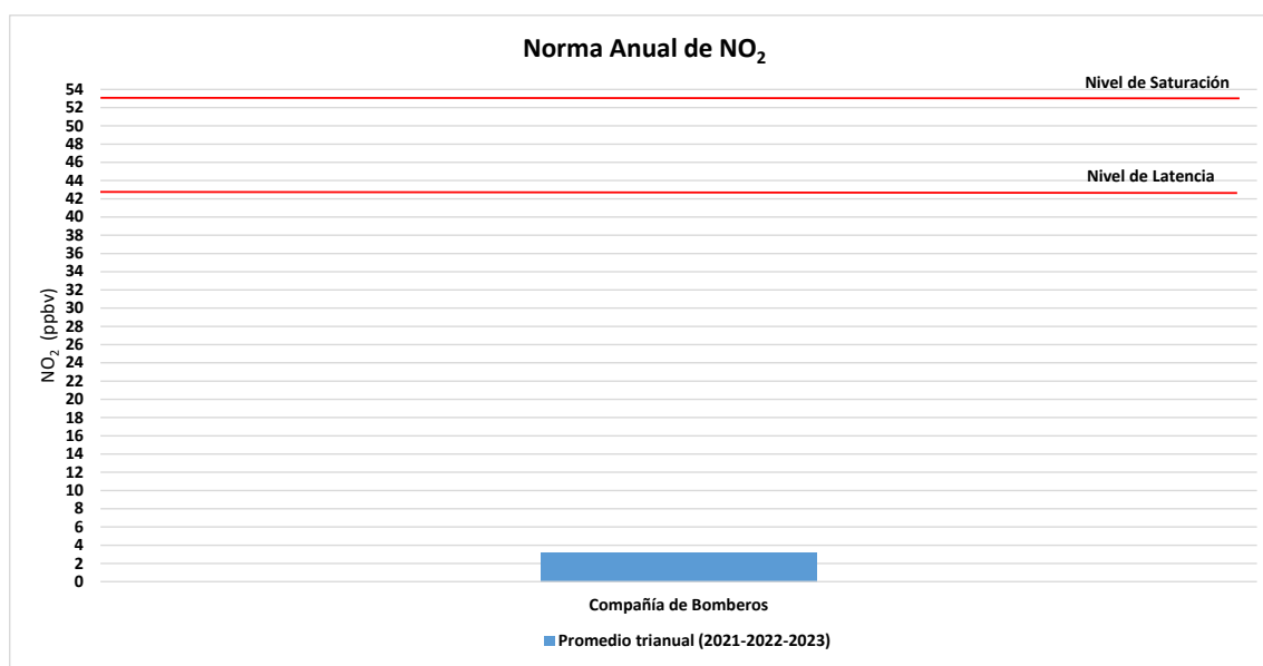
Gráfico 4 Norma anual para NO 2 , promedio trianual para el período 2021 al 2023
