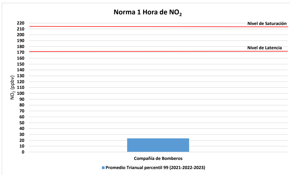
Gráfico 3 Norma 1 hora para NO 2 , promedio trianual para el período 2021 al 2023
