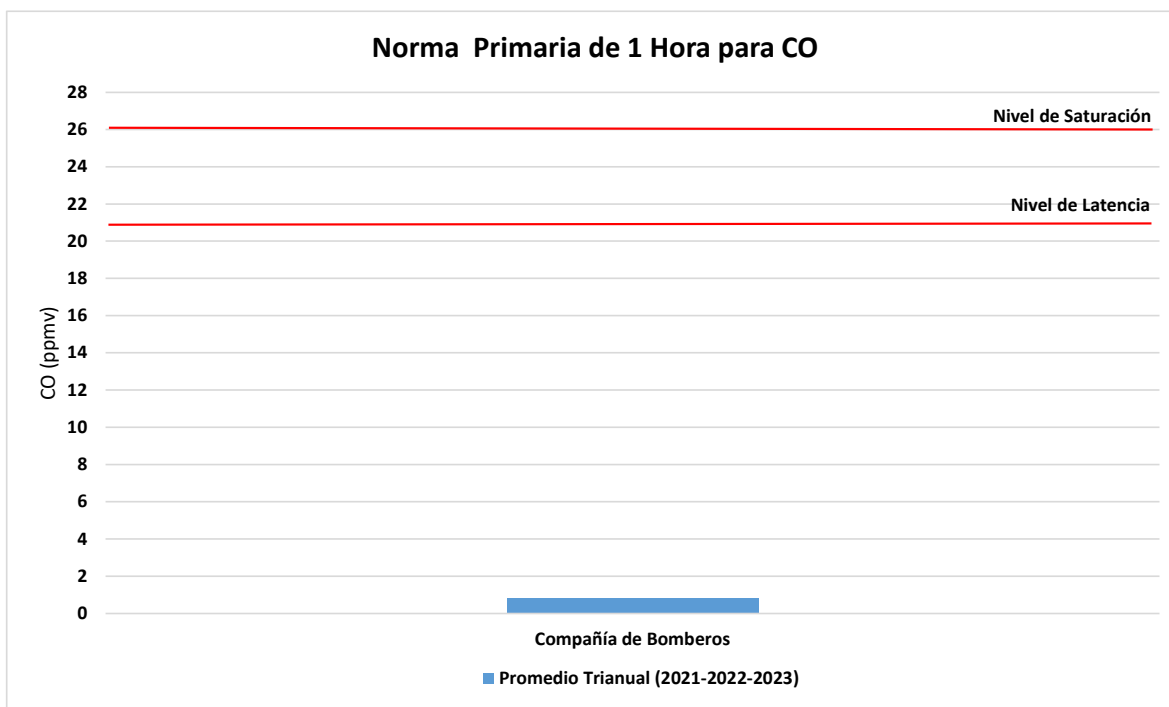
Gráfico 5 Norma 1 hora para CO, promedio trianual para el período 2021 al 2023
