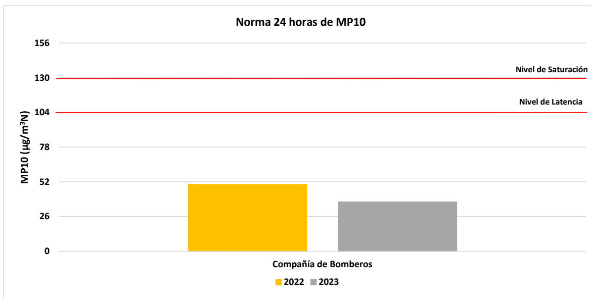
Gráfico 1 Norma 24 horas para MP10 para el año 2022 y 2023
