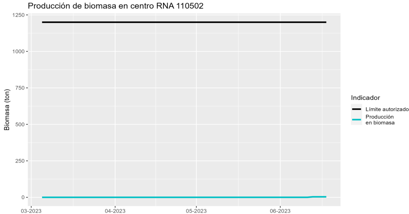
Figura 2. Producción de CES CHAFFERS 2 (RNA 110502) en todos los ciclos analizados
