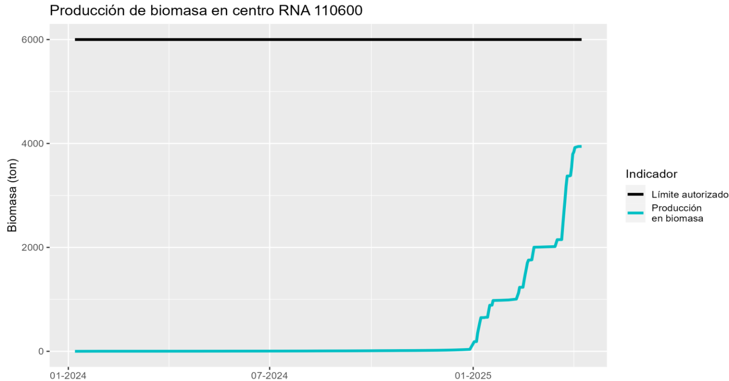
Figura 2. Producción de CES BENJAMIN (RNA 110600) en todos los ciclos analizados
