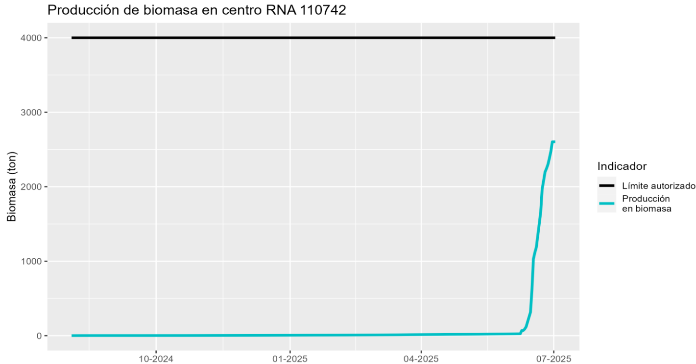
Figura 2. Producción de CES BAHIA ANITA (RNA 110742) en todos los ciclos analizados
