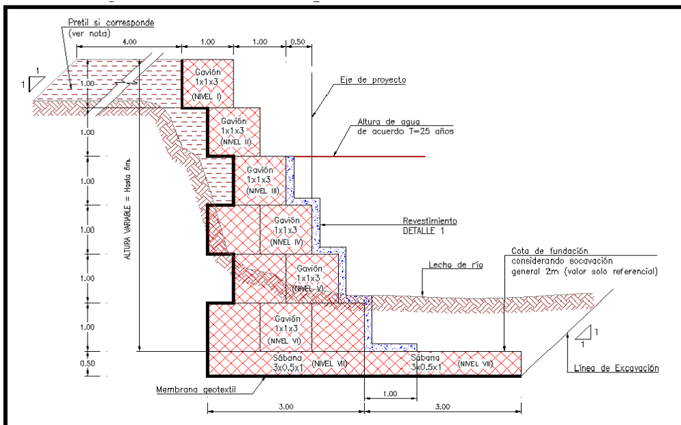
Figura N°1. Protección Fluvial tipo del Proyecto.
