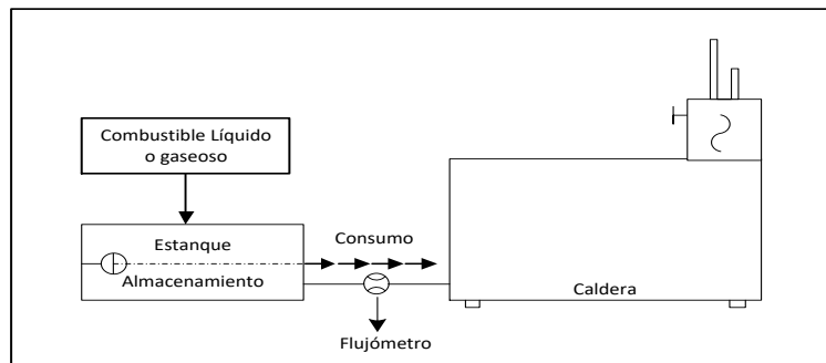
Figura 3 – Caldera con combustible líquido y/o gas.
