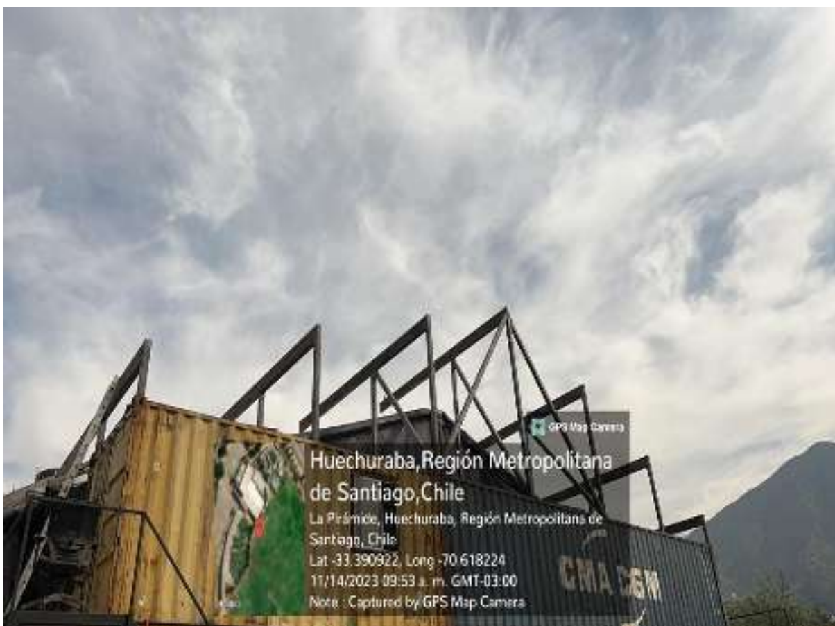
Vista posterior de la barrera perimetral acústica de dos niveles con techumbre en voladizo
