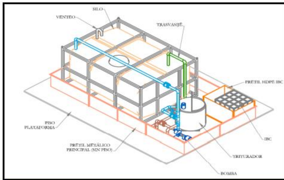
Figura 1: Esquema de unidad de ensilaje y acopio.
