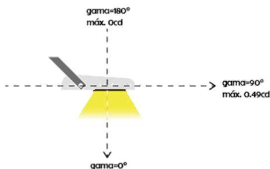
Ilustración 1. Representación de ángulo gama 90°
