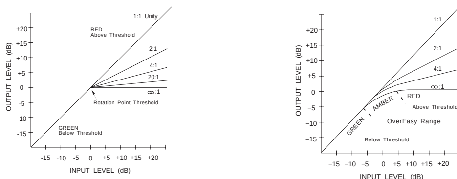
Figura 2: Curva de compresión con código inflexible, curva de compresión OverEasy® y LEDs de umbral
