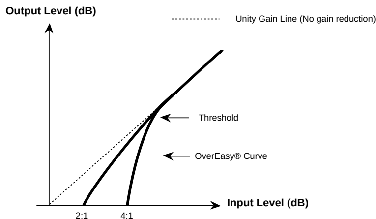
Abb. 1: OverEasy®-Kennlinie der Expander/Gate-Funktion
