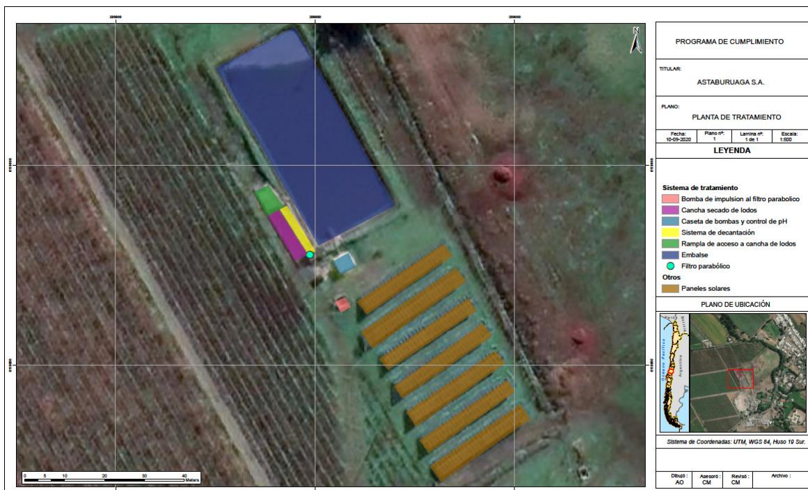
Imagen 1. Plano lay-out de las unidades correspondientes al sistema de tratamiento de Riles de Viña Astaburuaga, de 10 de septiembre de 2020
