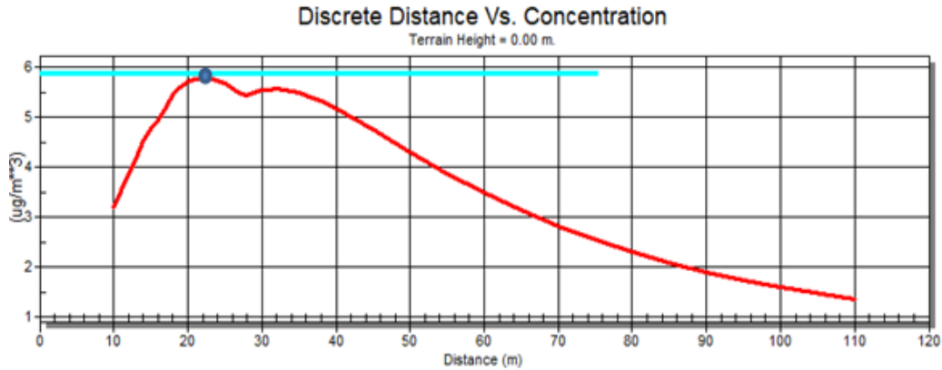
Figura 1. Distribución de las emisiones atmosféricas modeladas para 1 calefactor.
