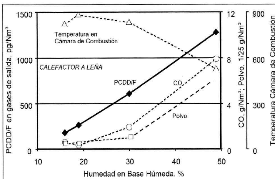
Emisiones de un calefactor v/s humedad de la leña
