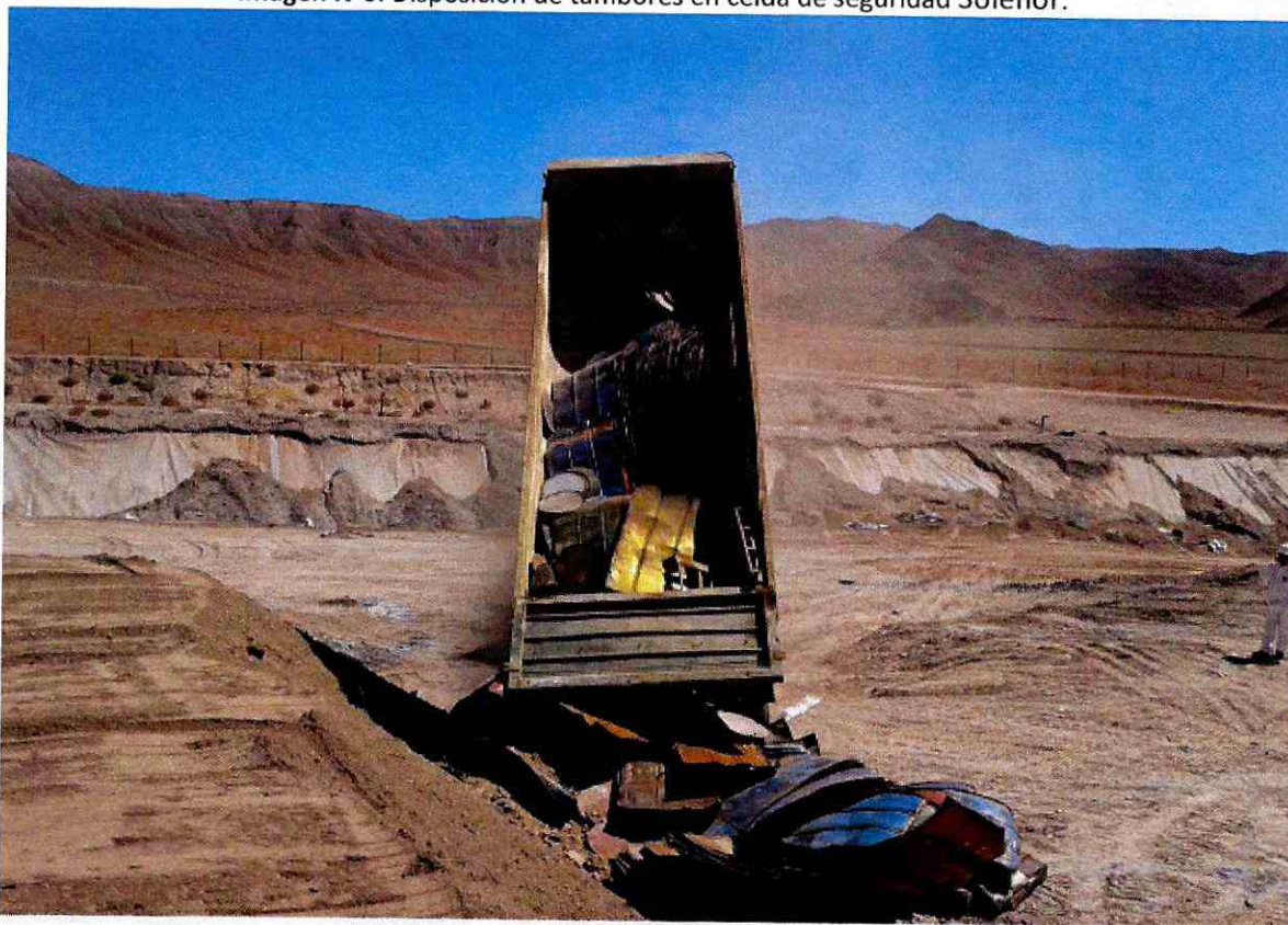
Imagen N°6: Disposición de tambores en celda de seguridad Solenor.
