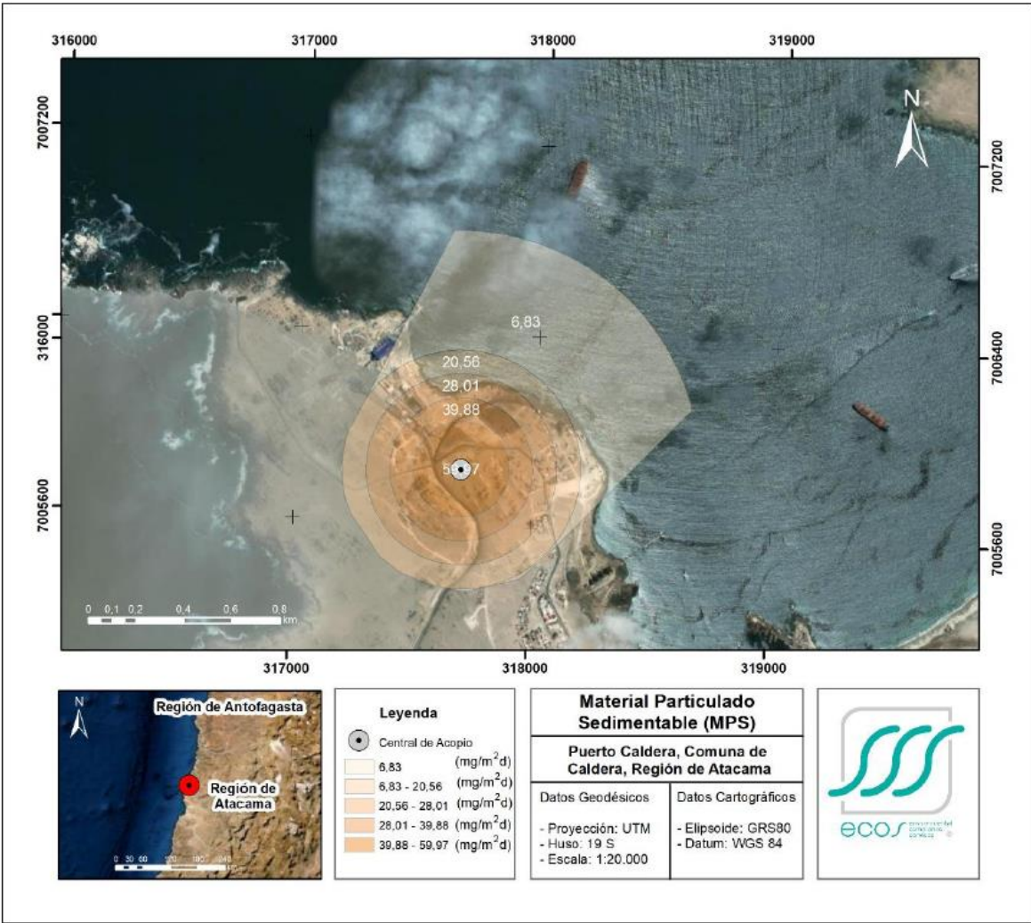
Figura 13. Isoconcentraciones de MPS desde la fuente emisora
