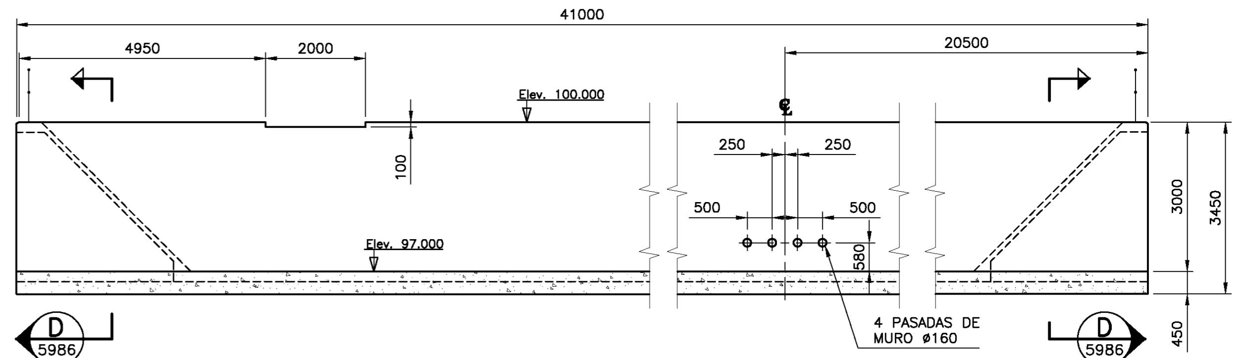
CORTE B Esc. 1 : 75
