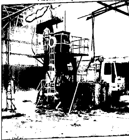
Fotografía - 8 Piscina de separación
