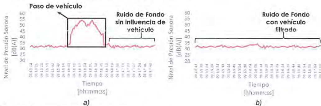
Figura 4. Gráfico de: a) una medición con la influencia del paso de un vehículo y b) misma medición filtrando el paso del vehículo.
