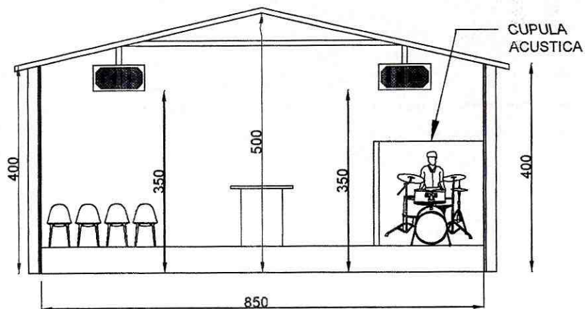
ELEVACION ALTAR ESCALA 1:100
