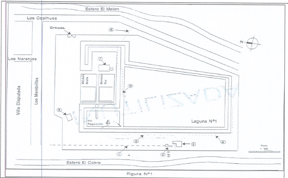
Figura 2.1 Diagrama esquemático de operaciones unitarias de la Planta de Tratamiento El Melón. Fuente: Figura N° 1 Declaración de Impacto Ambiental.
