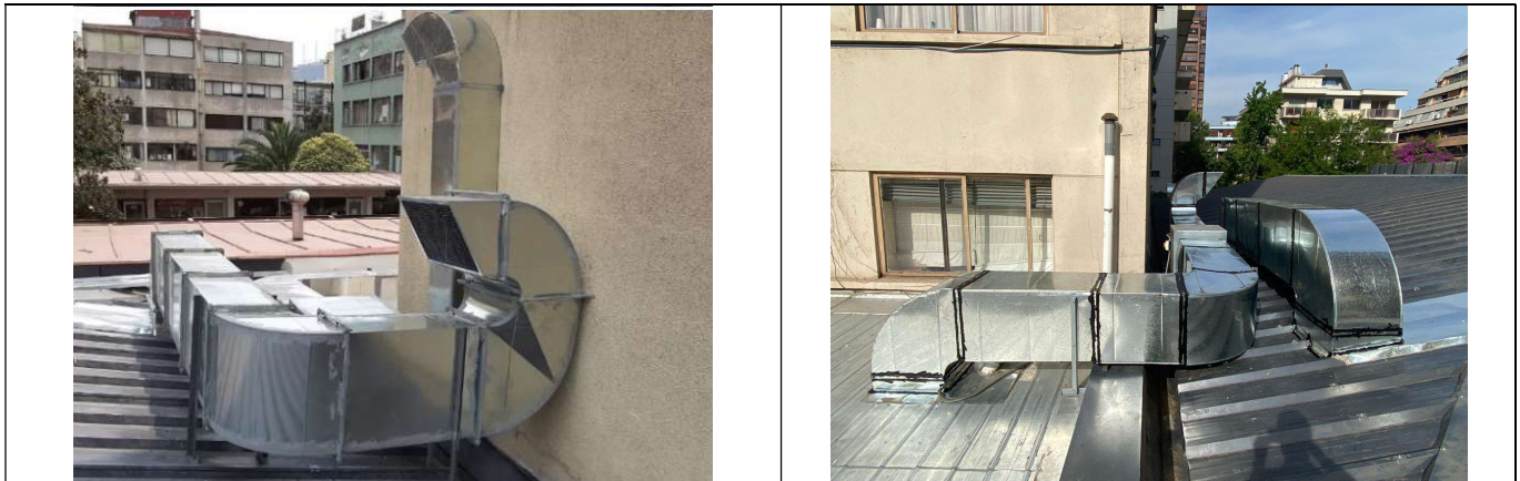
Aislación y modificación de ductos de inyección y extracción del local
