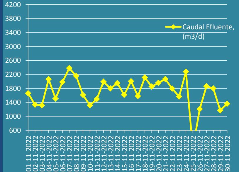
Caudal Efluente , Noviembre 2022 (m3/d)
