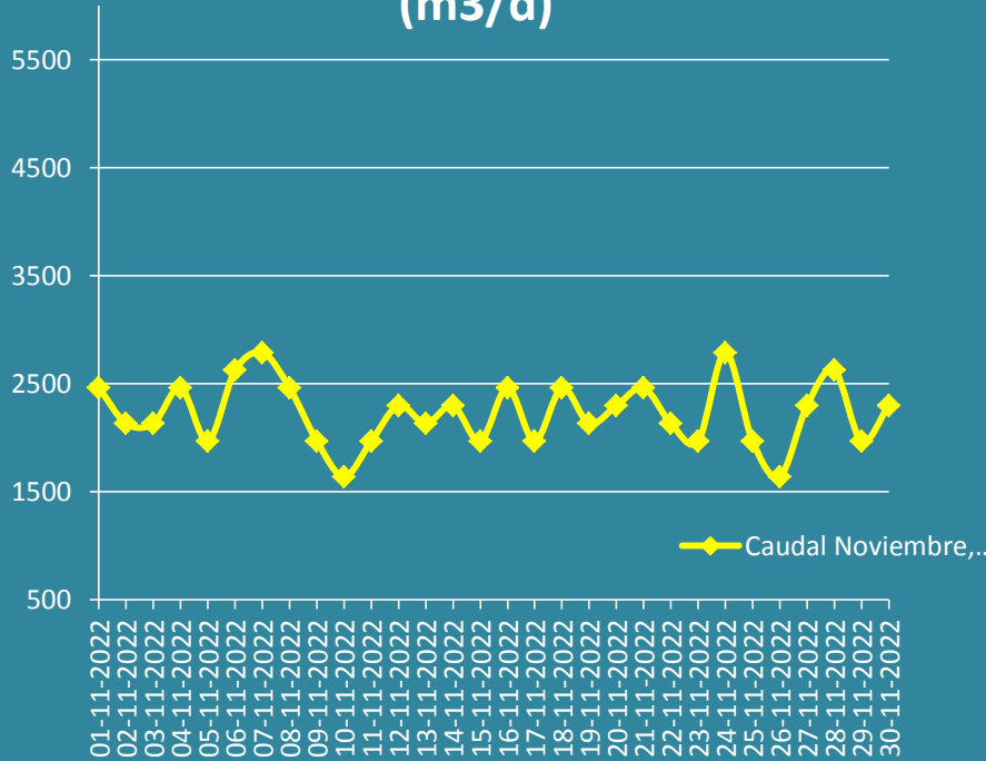
Caudal Afluyente ,Noviembre 2022 (m3/d)
