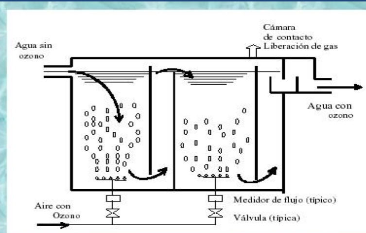
CÁMARA DE CONTACTO CON DEFLECTORES
