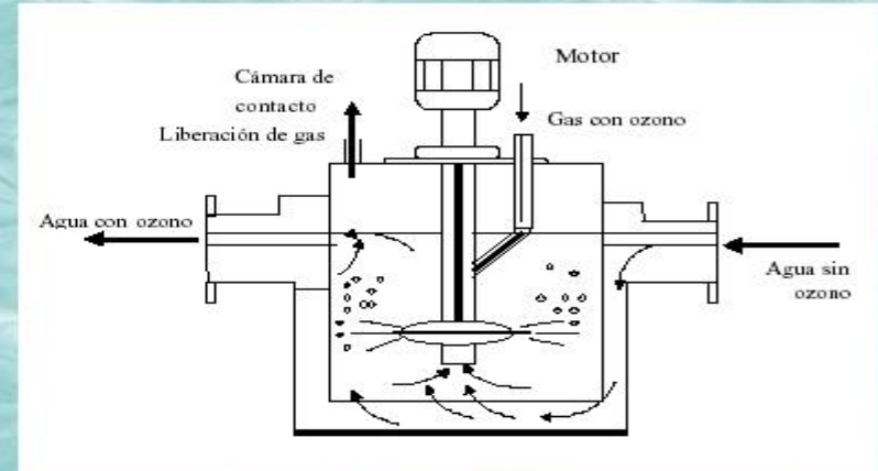
DIFUSOR DE TURBINA
