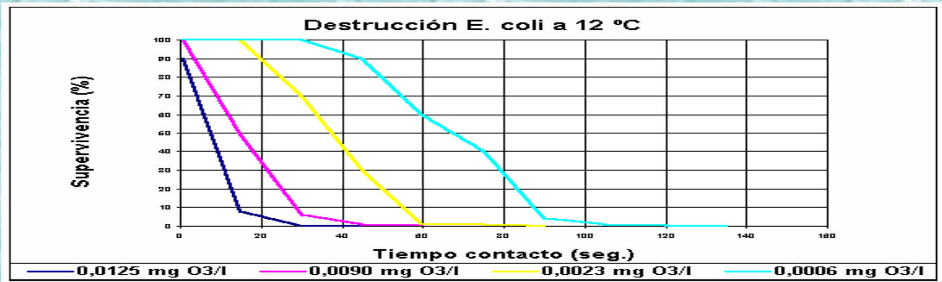
ACCION DEL OZONO SOBRE E.COLI
