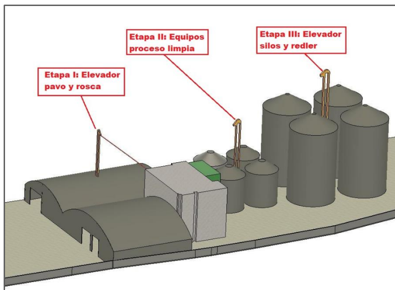
Modelamiento de la planta y sus equipos.
