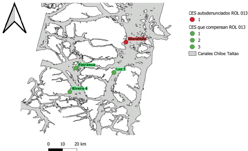
Figura 1: Mapa de distribución geográfica de los CES autodenuncias y CES compensatorios, correspondientes al Rol A-013-2023. Fuente: Anexo 1 del Informe “Análisis de la Idoneidad Ecosistémica del Plan de Compensación en el marco de la Autodenuncia por la sobreproducción del Grupo Australis”.
