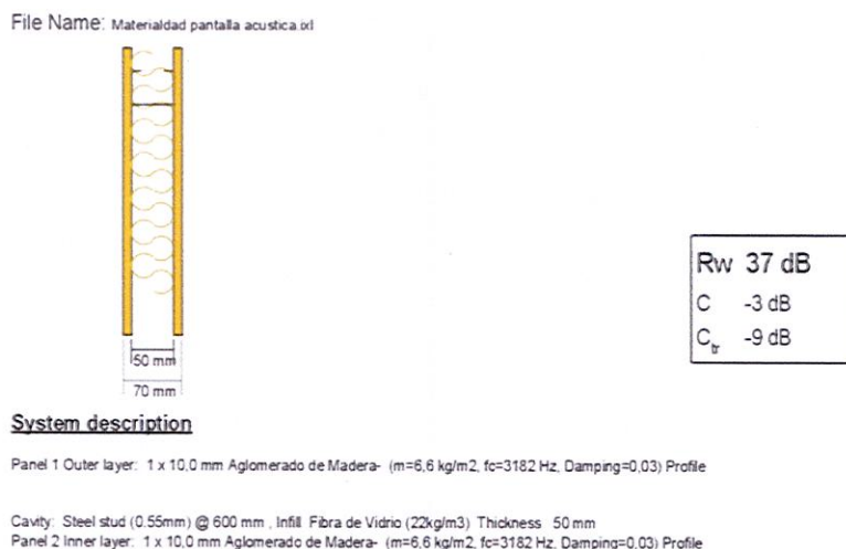
Figura 13. Materialidad de pantalla acústica.
