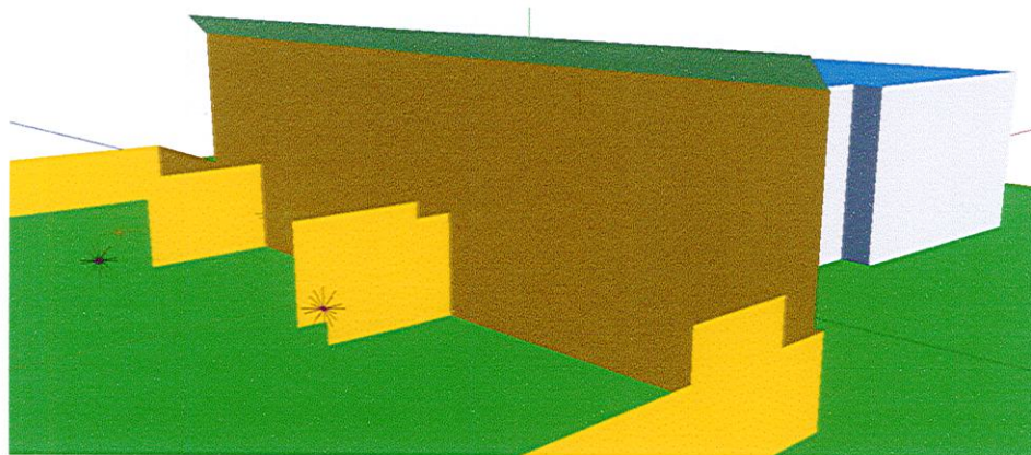
Figura 12. Pantalla acústica de 7 m de altura más pantalla inclinada de 1 m.
