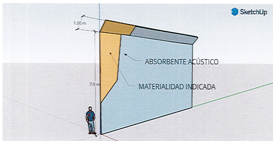
Figura 14. Dimensiones de pantalla acústica.
