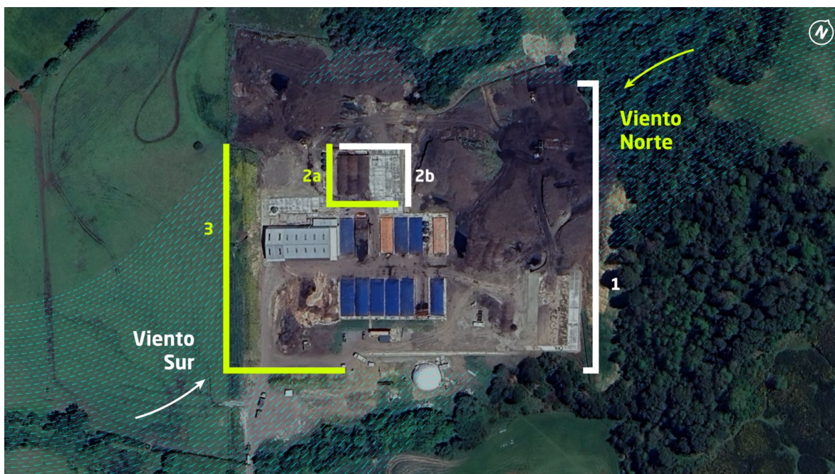
Figura 1: Líneas de aspersores de la planta
