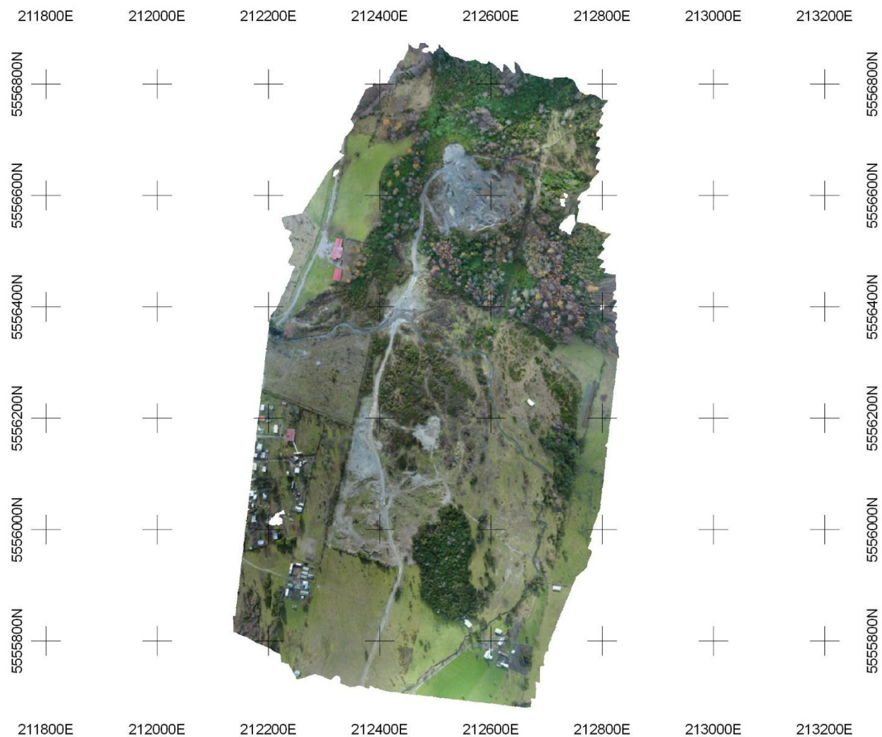
Figura 2. Layout del proyecto (Pozos de extracción de áridos)
