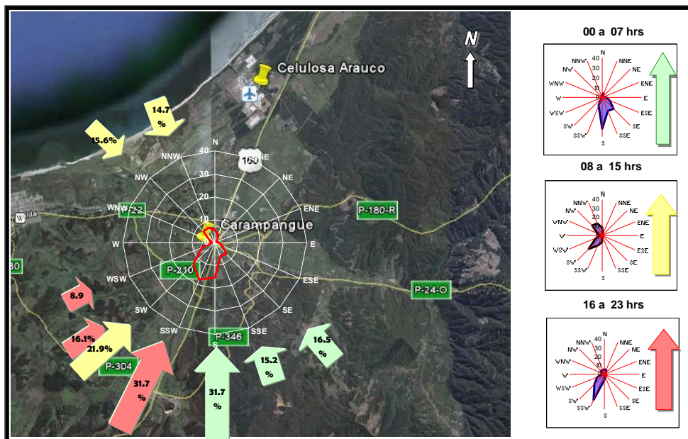
FIGURA 4.1.2: ROSA DE VIENTO ESTACIÓN CARAMPANGUE, FEBRERO DE 2013
