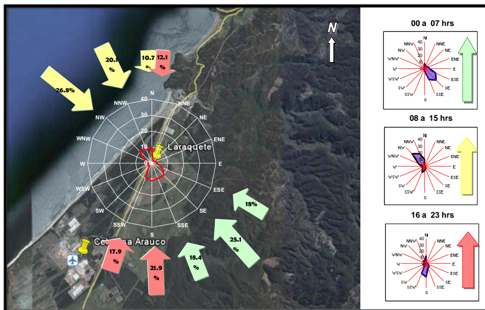
FIGURA 4.2.2: ROSA DE VIENTO ESTACIÓN LARAQUETE, FEBRERO DE 2013
