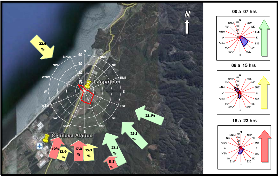
FIGURA 4.2.3: ROSA DE VIENTO ESTACIÓN LARAQUETE, MARZO DE 2013
