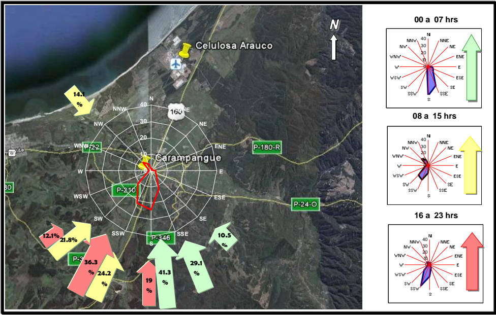
FIGURA 4.1.3: ROSA DE VIENTO ESTACIÓN CARAMPANGUE, MARZO DE 2013
